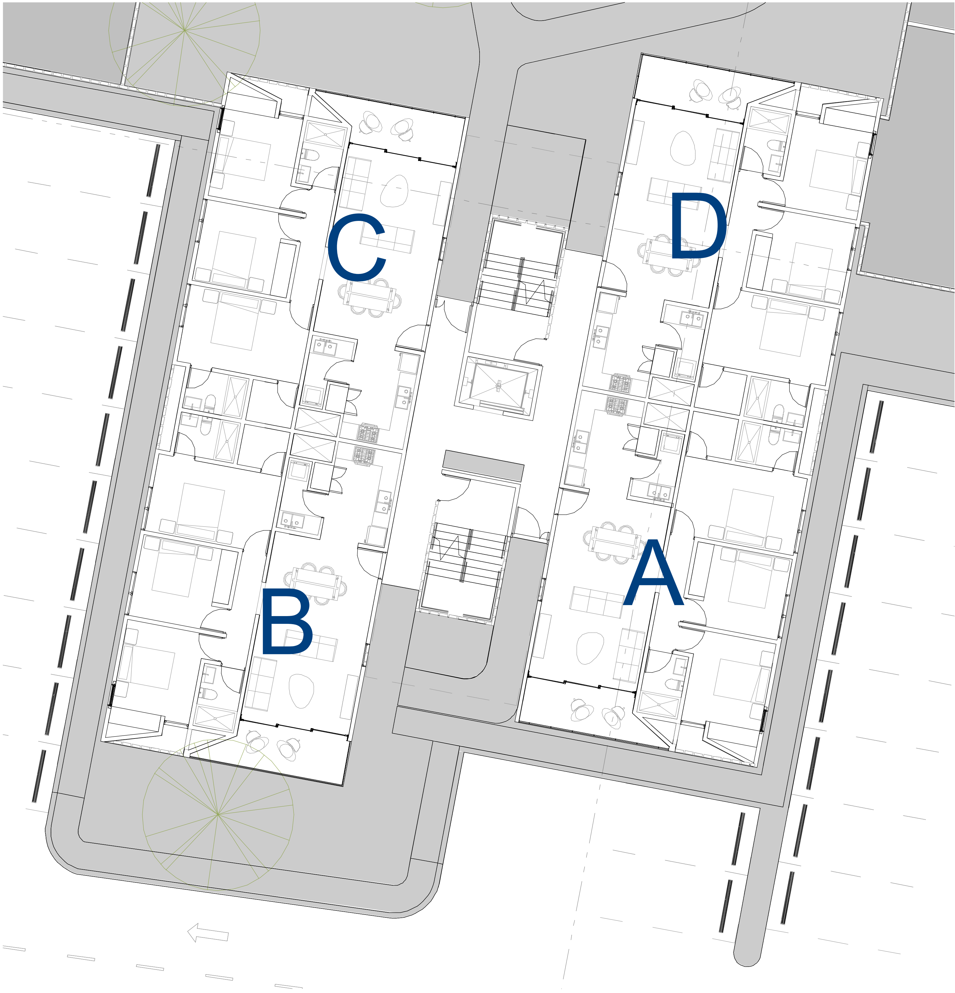
1 PLANTA ARQUITECTÓNICA Niv 1 al Niv 8- Edif (2-4-6-7) 1 : 50
