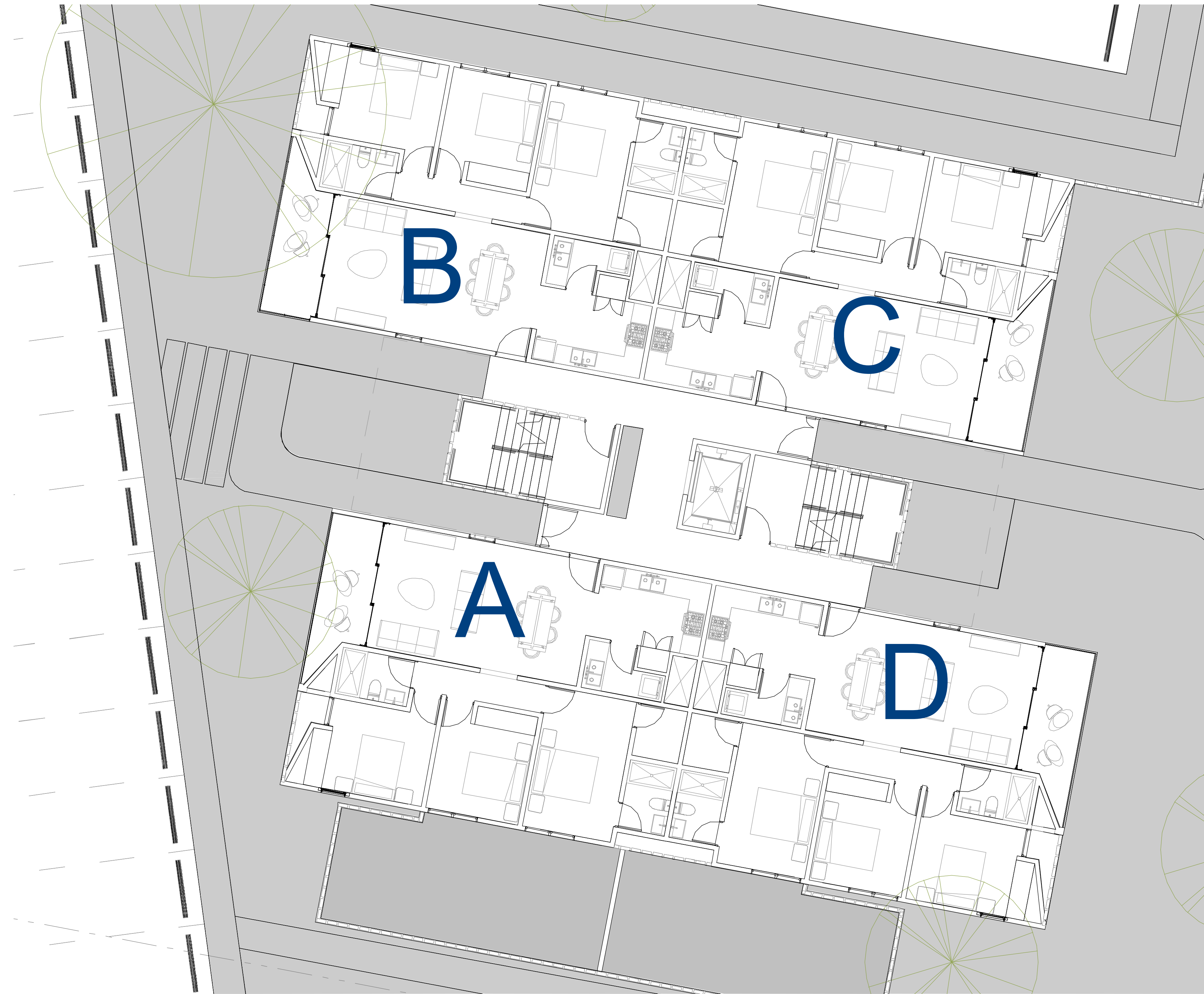
1 PLANTA ARQUITECTÓNICA Niv 1 al Niv 8- Edif (8) 1 : 50
